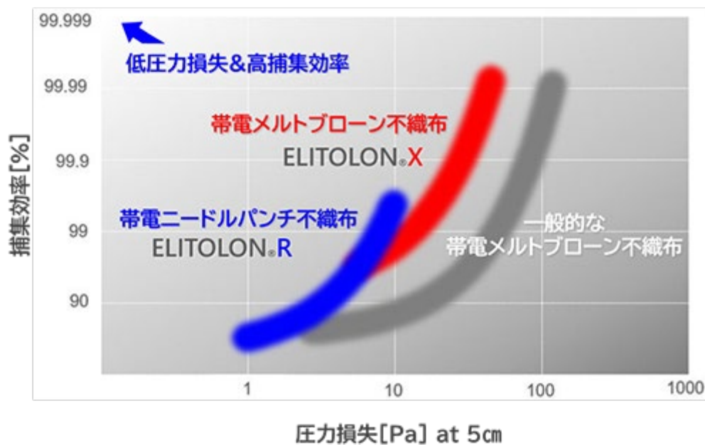
0.3μm粒子捕集効率と圧力損失
